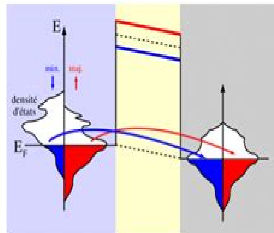
(b) Alignement anti-parallèle
