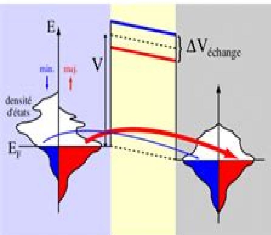
(a) Alignement parallèle
