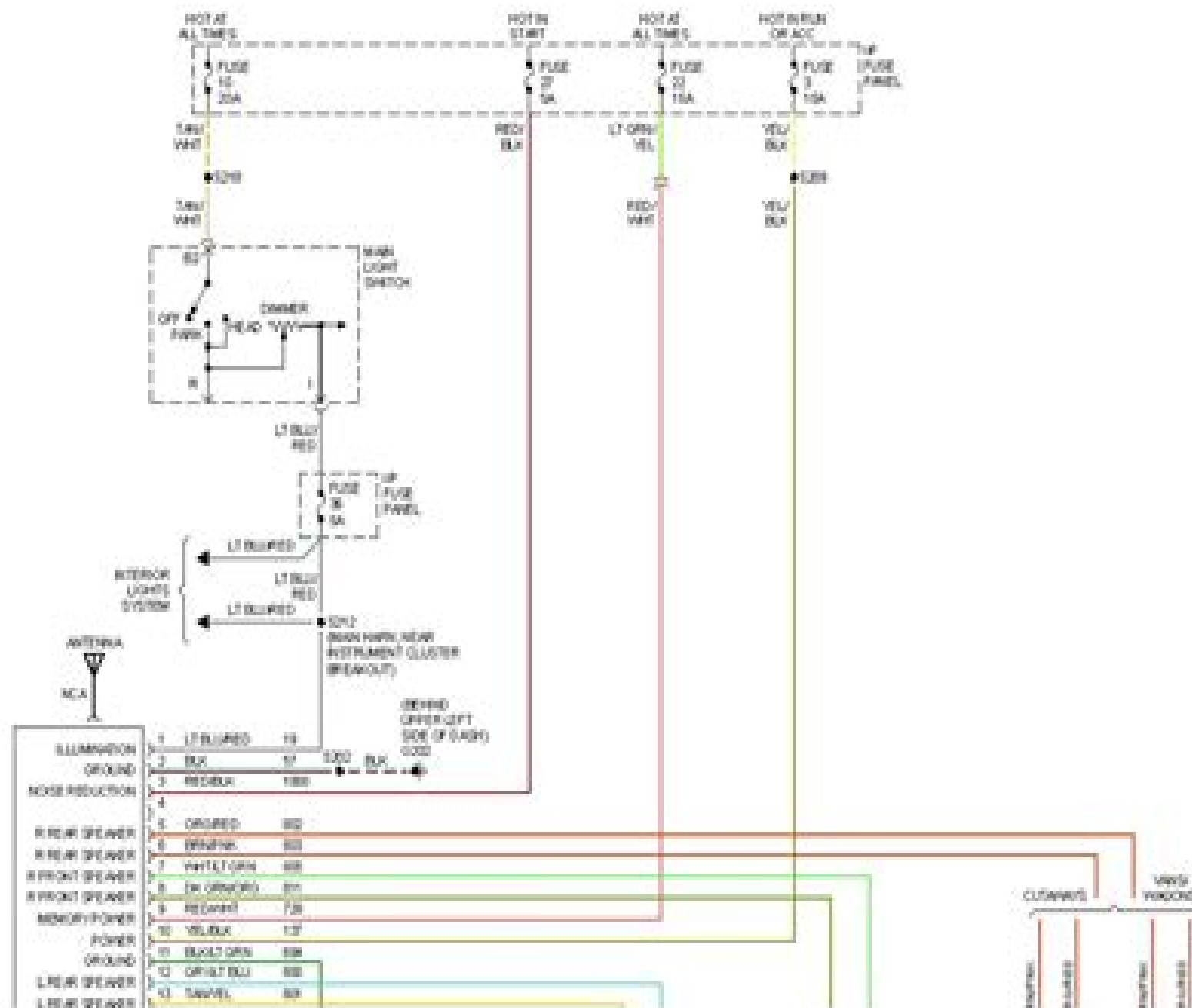
1998 Ford Econoline E350-Fig. 59: Radio Circuits
