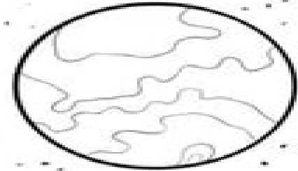
VENUS
