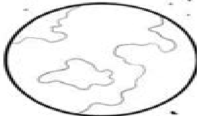
SUN
