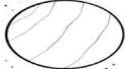
URANUS
