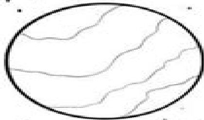
MARS
