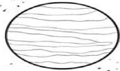
JUPITER
