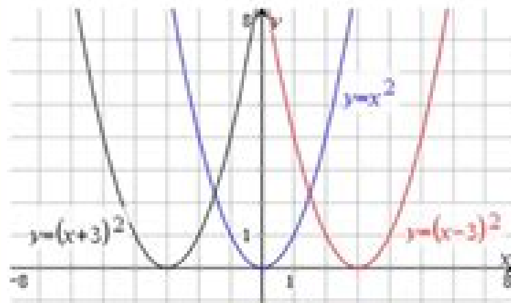
Horizontal Shift ( Left ) Horizontal Shift ( Right )
