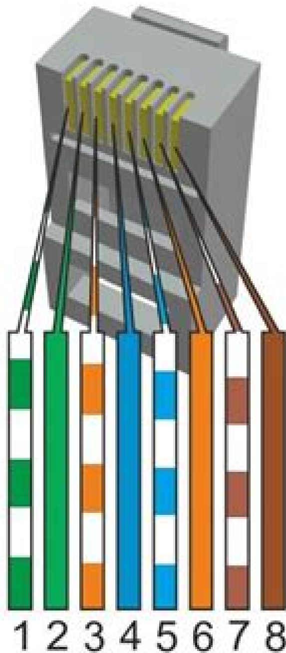
T-568A
