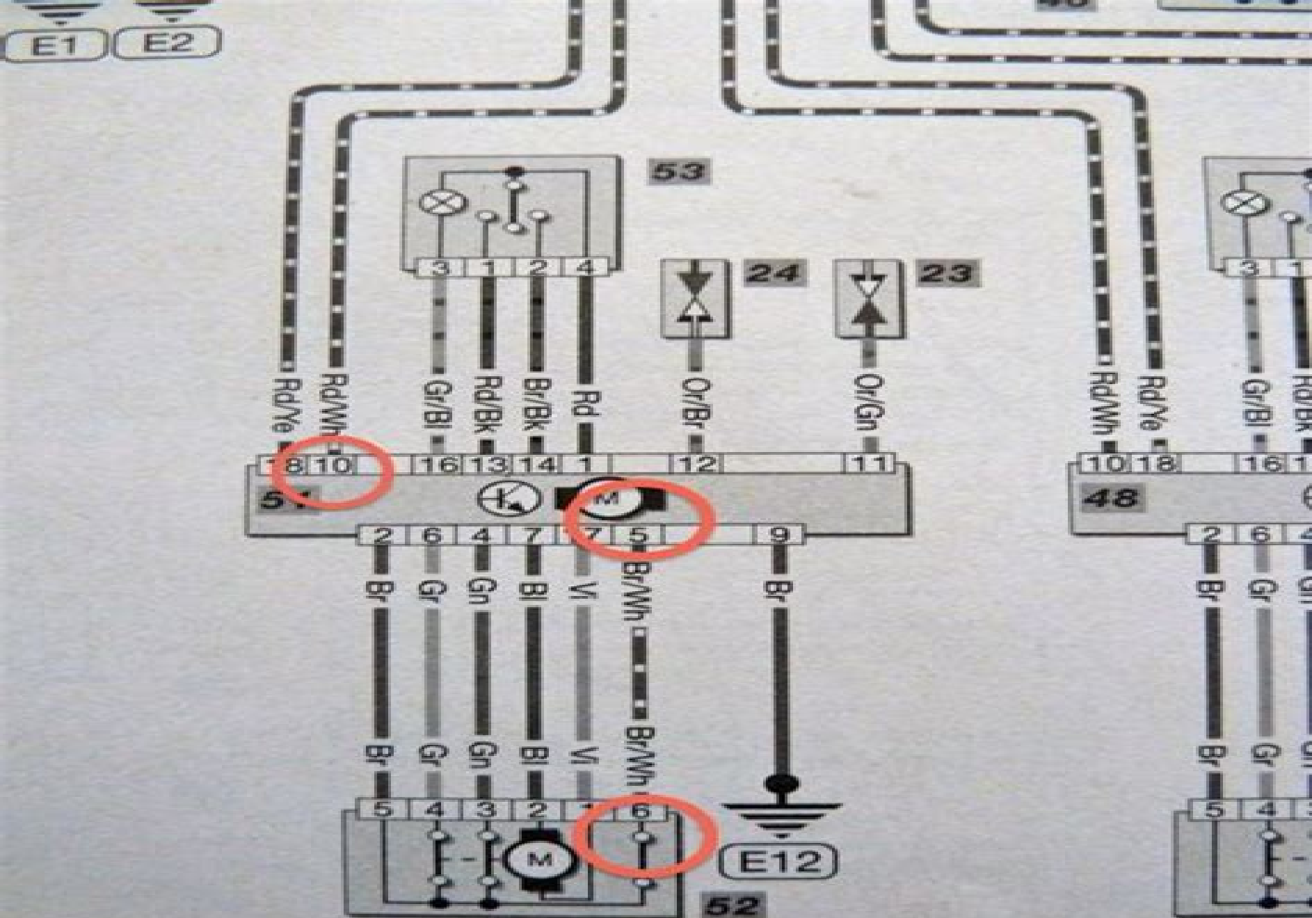
51: WindowMotor / 52: DoorLock
