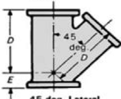
45 deg. Lateral
