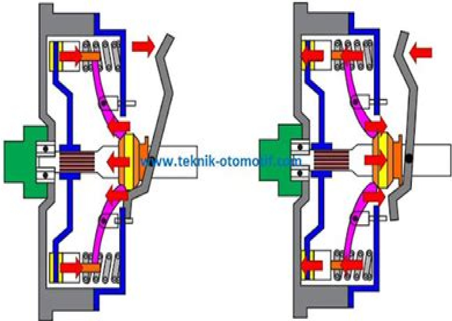
Saat Pedal Kopling Ditekan
