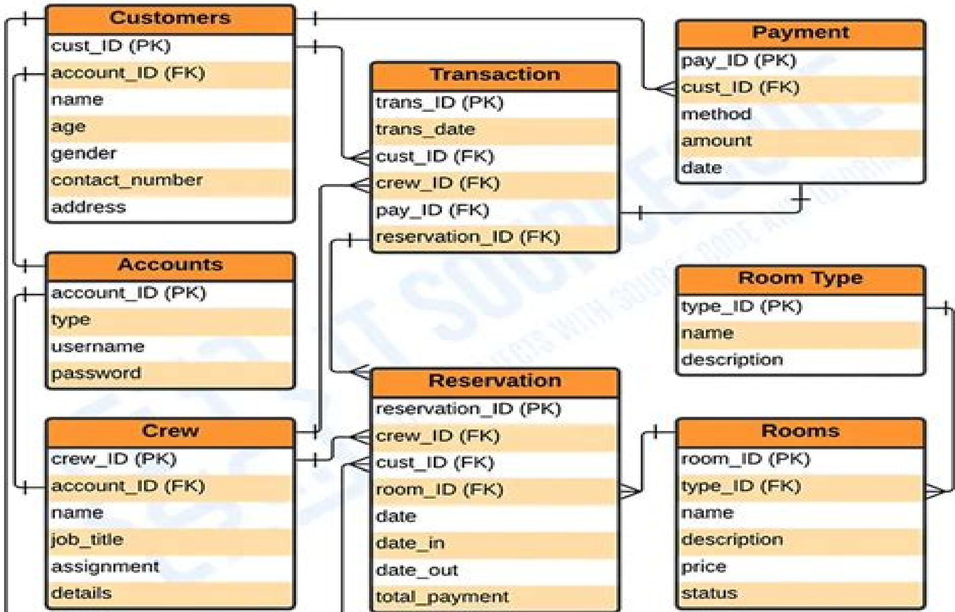
ER DIAGRAM
