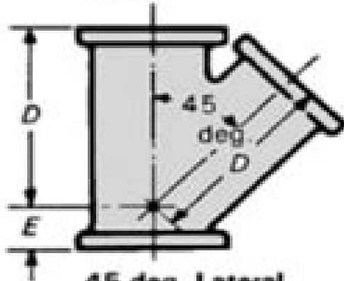
45 deg. Lateral
