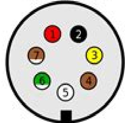
ISO 7638-1
