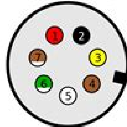
ISO 7638-2
