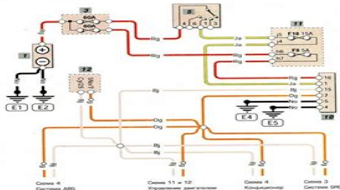
Диагностический разъем
