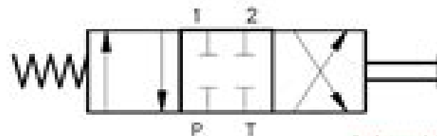
MANUAL ACTUATION
