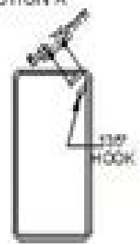
HOOPS/STIRRUPS
