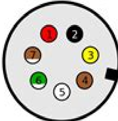
ISO 7638-2
