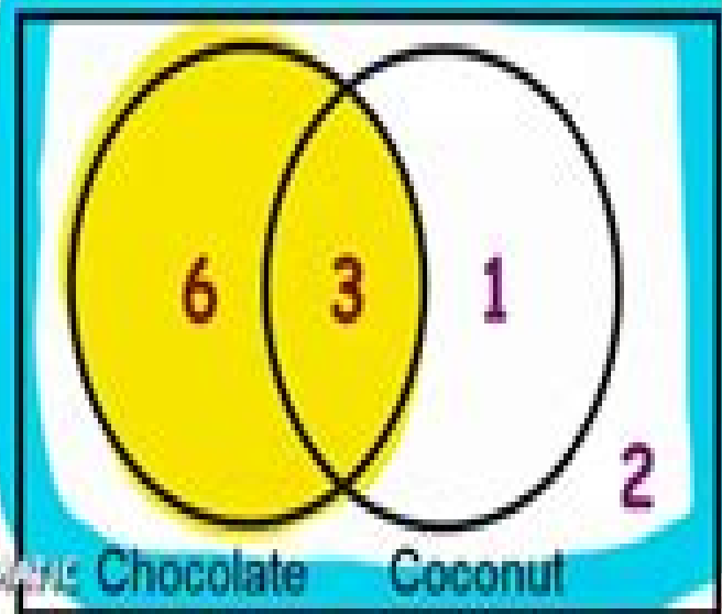
Venn Diagram
