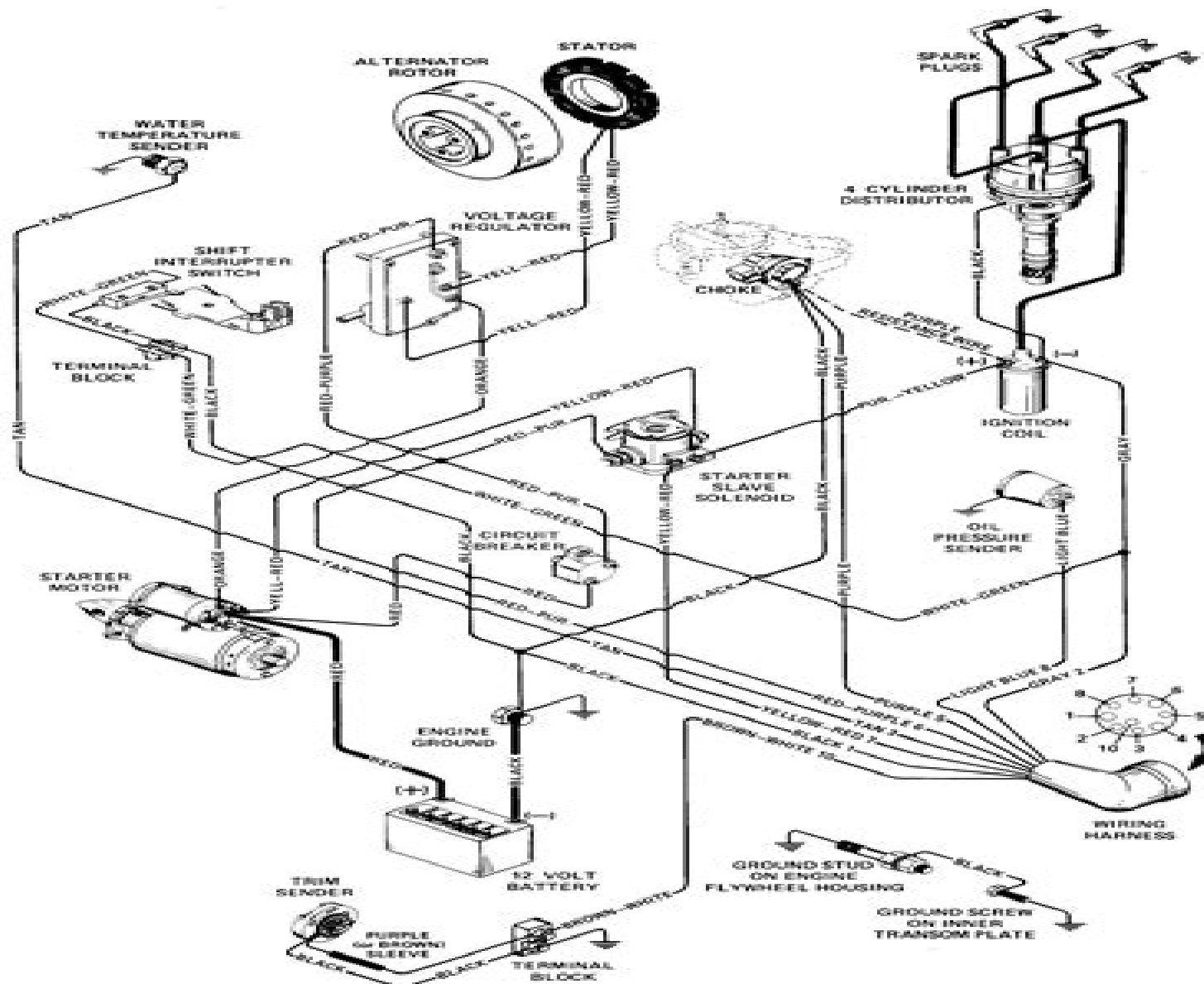
WIRING DIAGRAM 170/190
