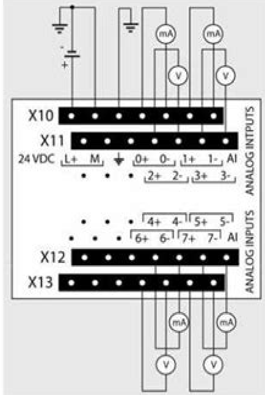
6ES7 231-4HF32-0XB0
