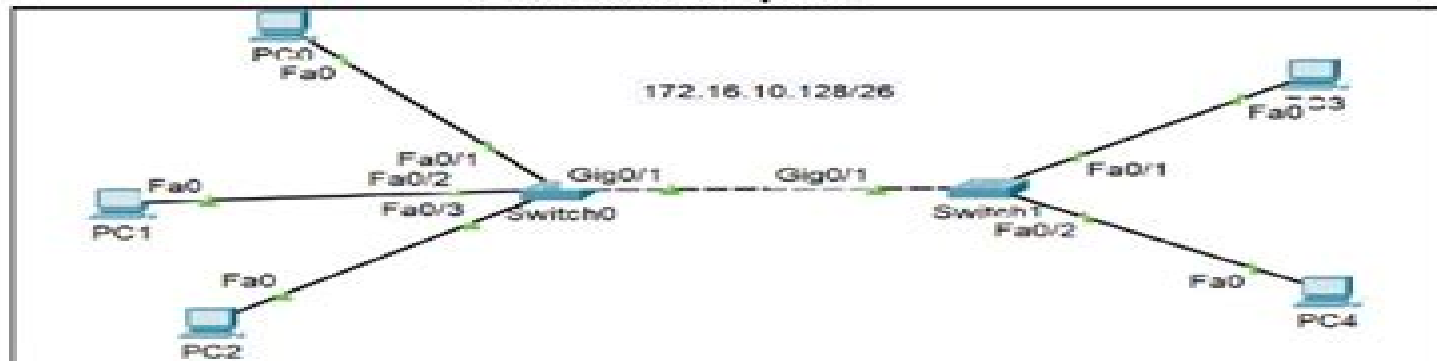
фиг. 1 LAN мрежа с два комутатора и пет крайни у-ва
