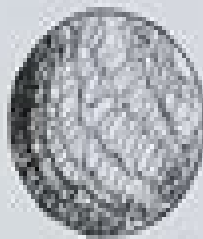
Scribbling
