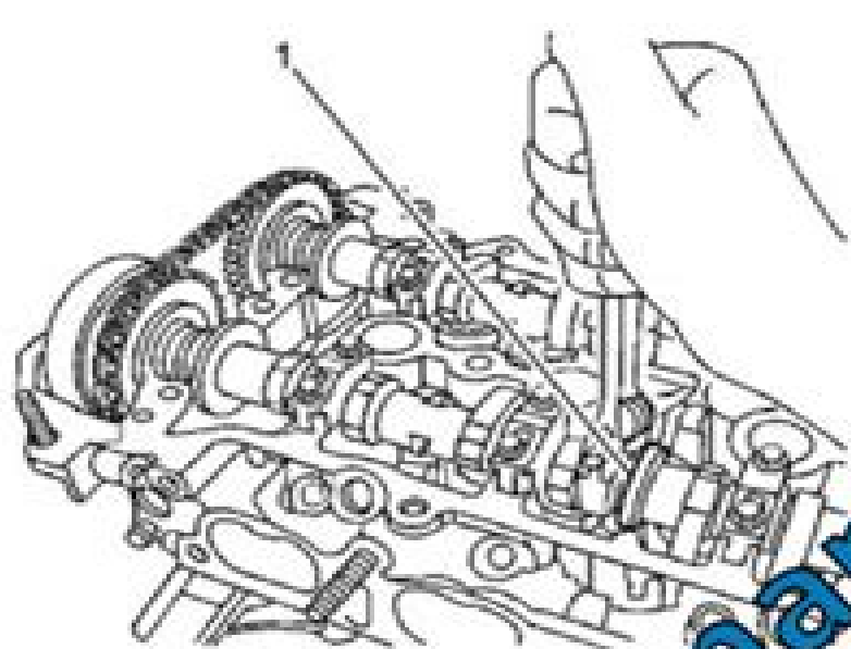
Fig. 109: Holding Camshaft
